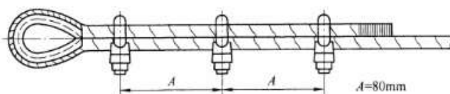
图 1 钢丝绳绳端固定
